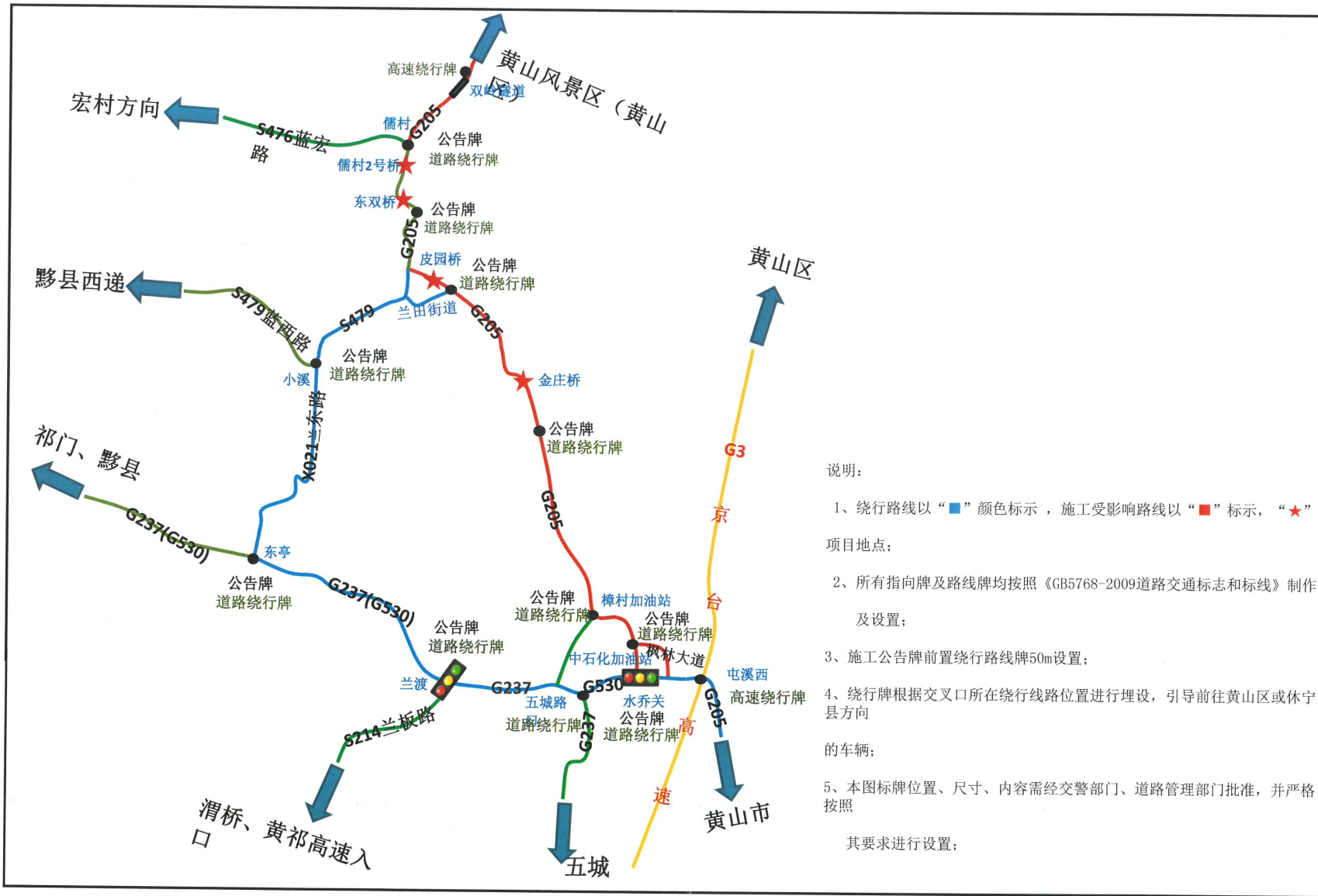
绕行路线标牌平面布置图
